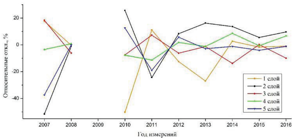
Рис. 4. Относительные отклонения кажущихся сопротивлений в различных слоях геоэлектрической модели в пункте 1P1
