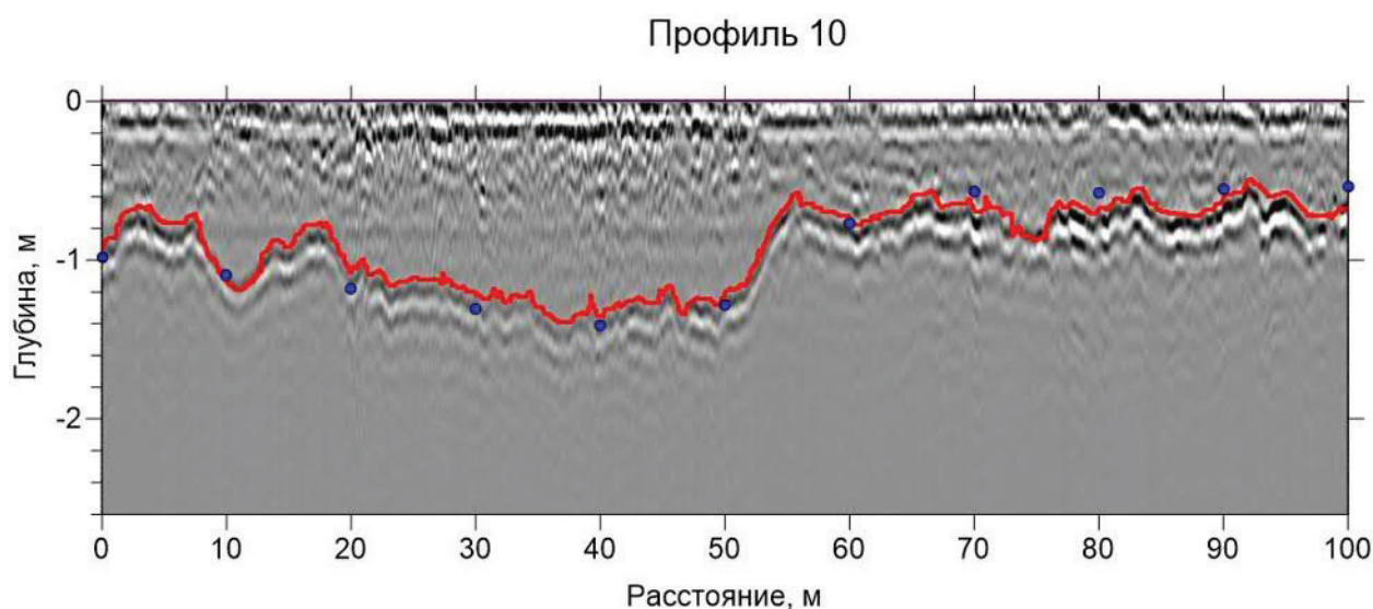
Рис. 1. Радарограмма и данные шупового опробования (синие точки)
